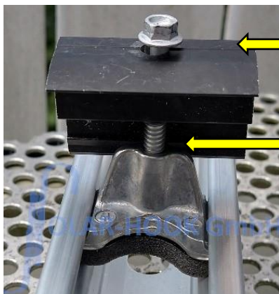
Abb. 14/ vormontierte Modul-Endklemme
